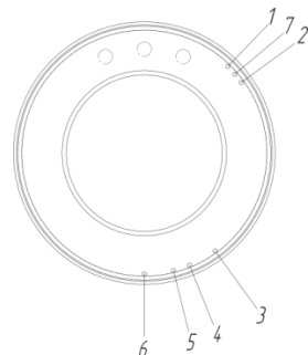
Рисунок 1. Расположение выводов
