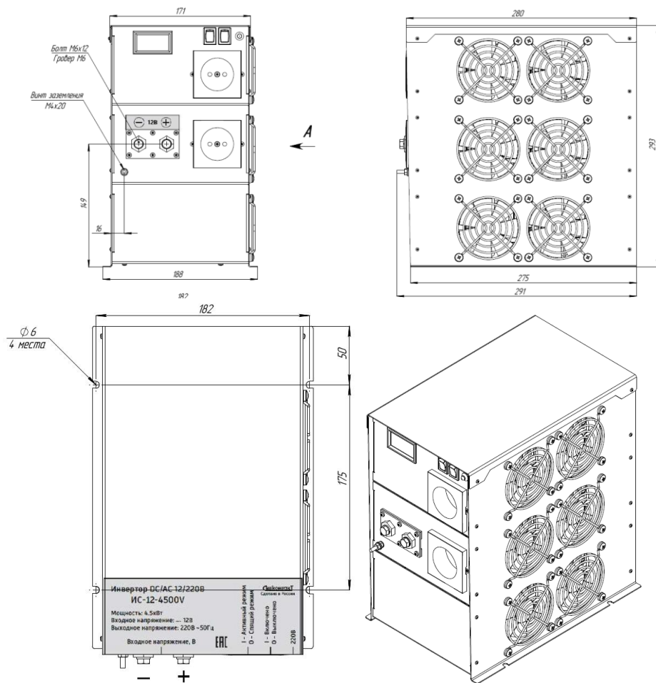
Рисунок 1.3- Внешний вид инвертора ИС-12-4500V.
