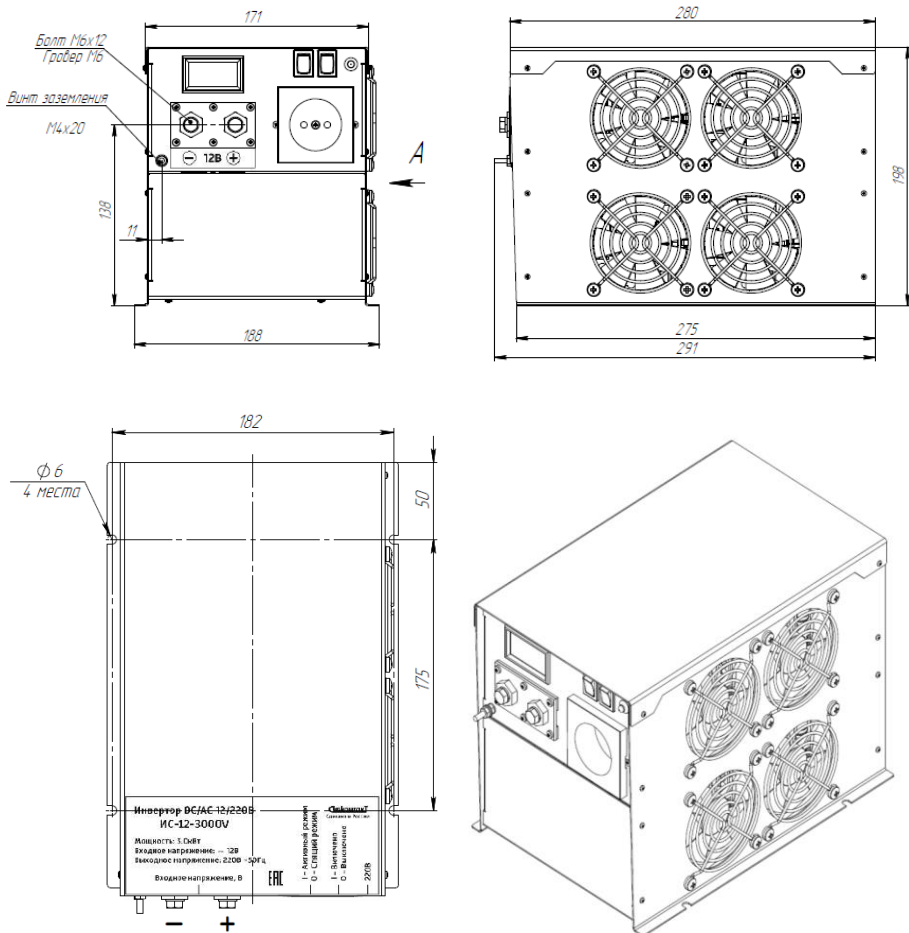
Рисунок 1.2- Внешний вид инвертора ИС-12-3000V.
