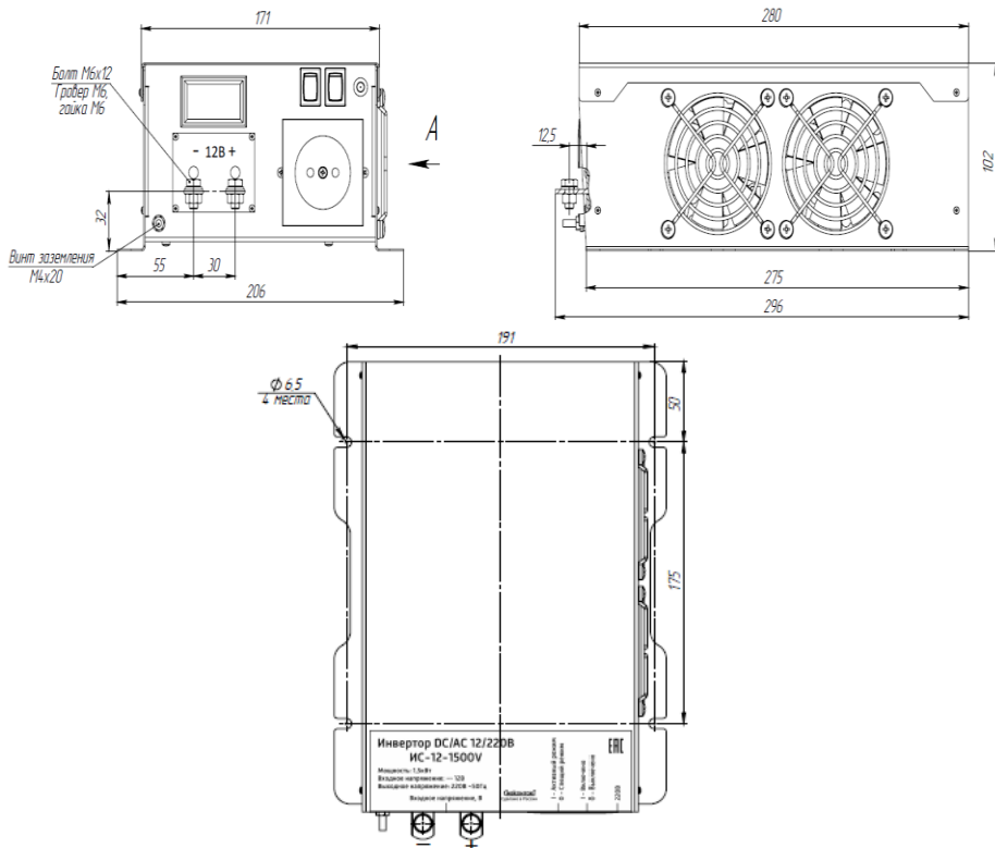
Рисунок 1.1- Внешний вид инвертора ИС-12-1500V.
